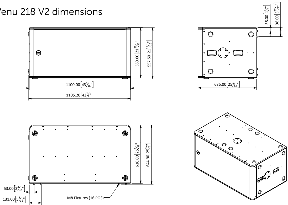
Figure B.12: Venu 218 V2 dimensions
