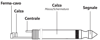
Uso sbilanciato del connettore jack TS 1/4"
