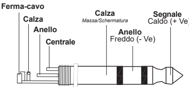
Uso bilanciato del connettore jack 1/4" TRS
